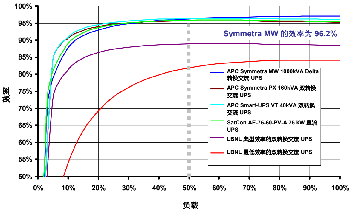
图 4 几种商用交流UPS 和直流UPS 系统的效率
